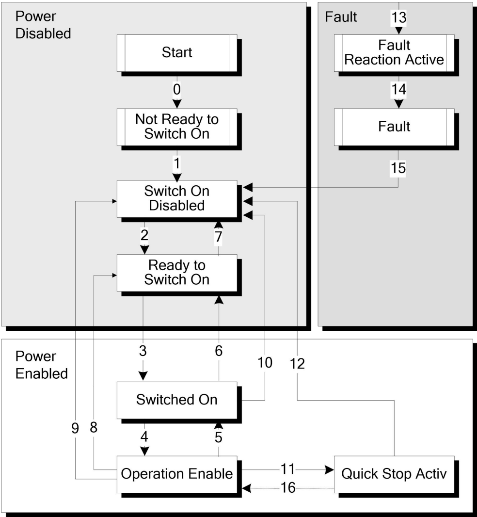
图 4-1CiA402 状态图
