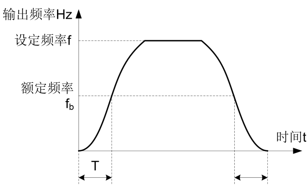
图 5-14 S 曲线加减速 B 示意
