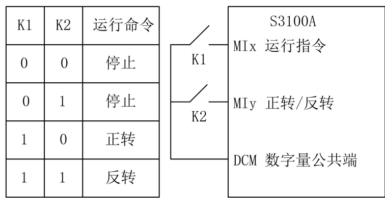
图 5-7 两线式模式 2
