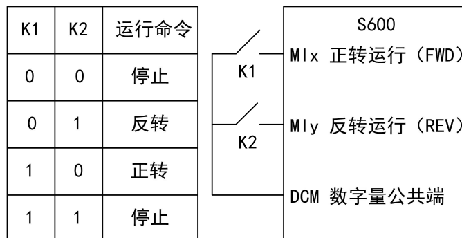
图 5-6 两线式模式 1
