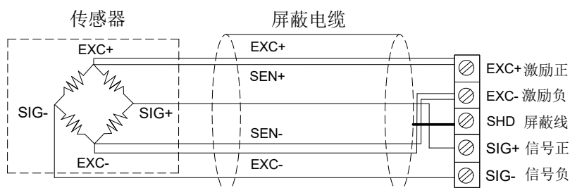
6 芯传感器与仪表接线图
