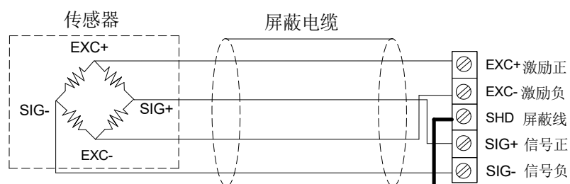
4 芯传感器与仪表接线图
