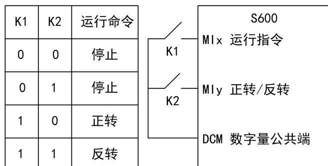
图 5-7 两线式模式 2
