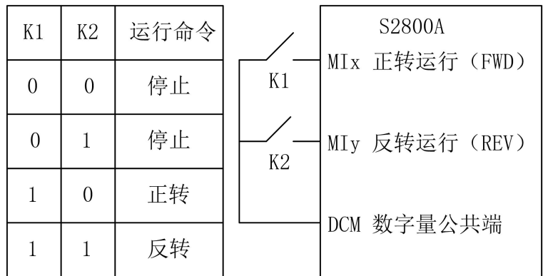
图 5-7 两线式模式 2
