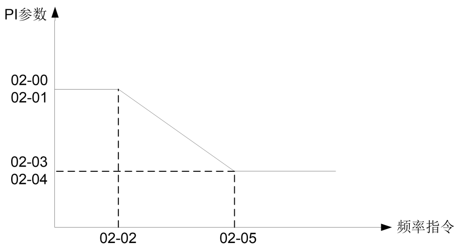
图 5-2 PI 参数示意图
