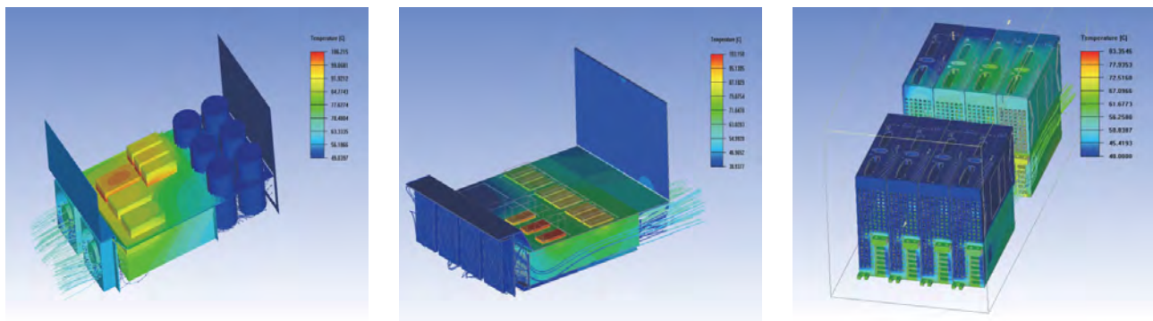
110kW变频器
