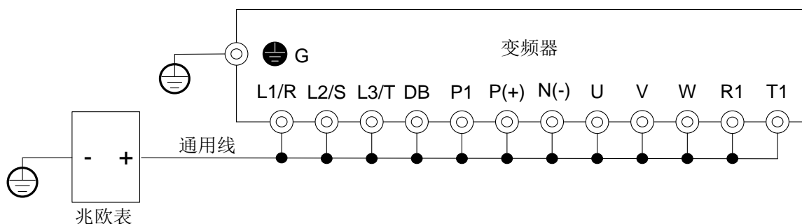
图 8.2 主回路绝缘电阻测试接线图
