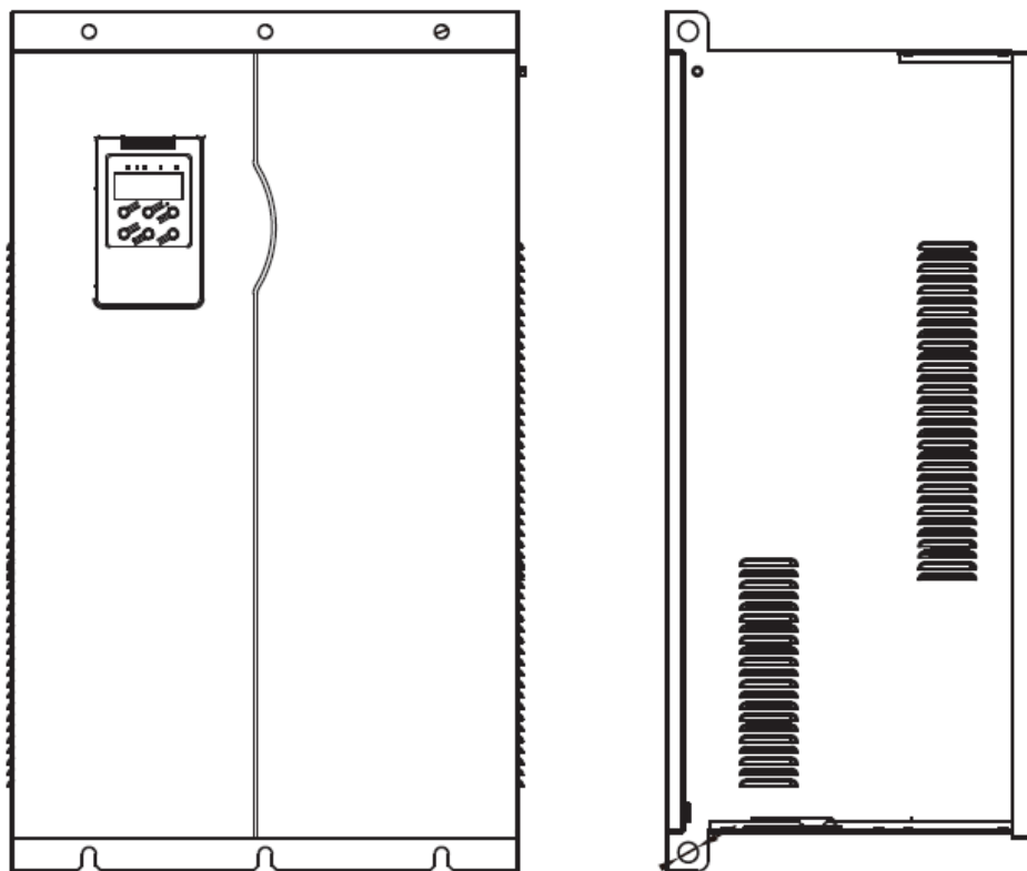
图 D (S5350-30kW~200kW 研发定形中)
