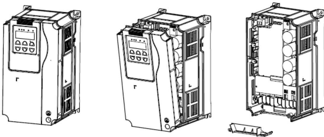
图 2.2 表面机盖与电缆引入板的拆卸(S5350-4T1.5G~22G 的情况)
