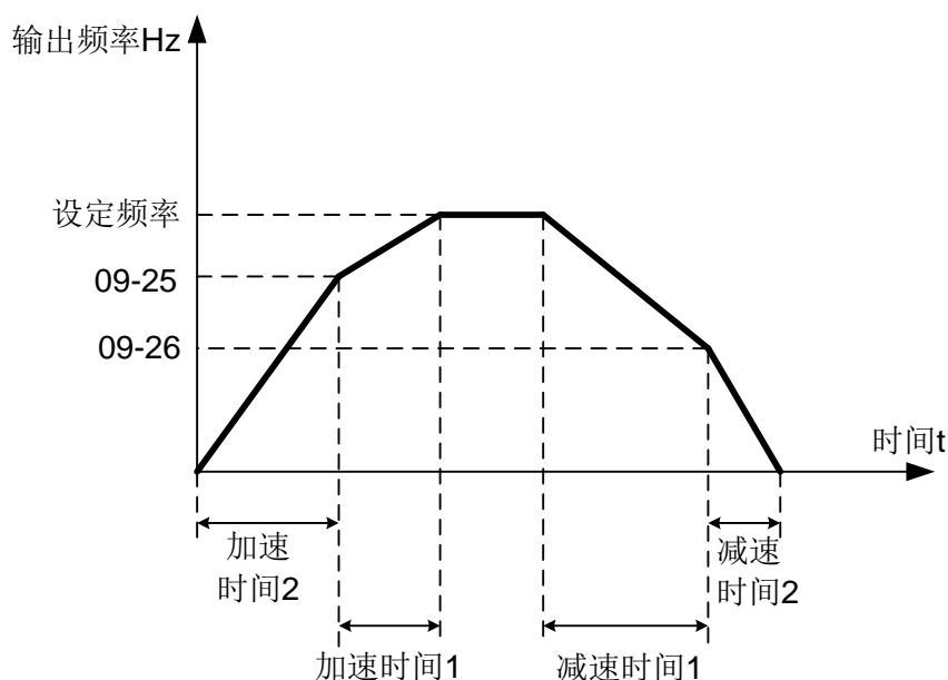
图 5-20 加减速时间切换示意图
