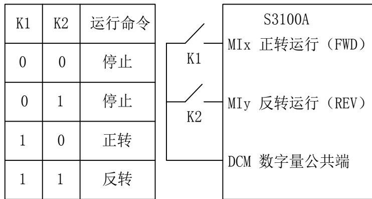
图 5-7 两线式模式 2
