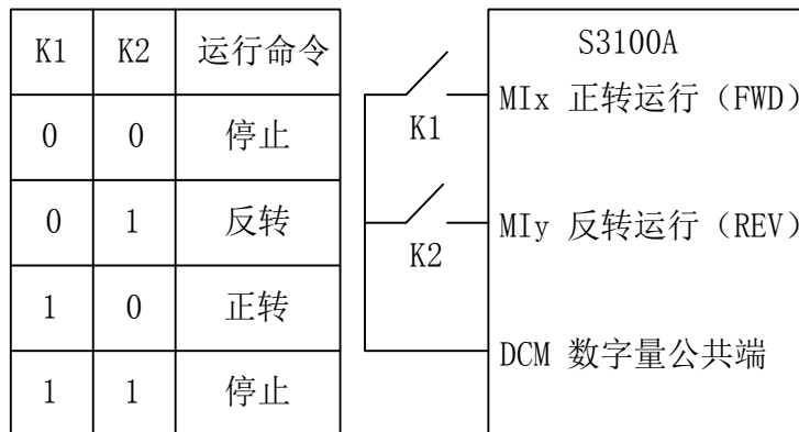
图 5-6 两线式模式 1
