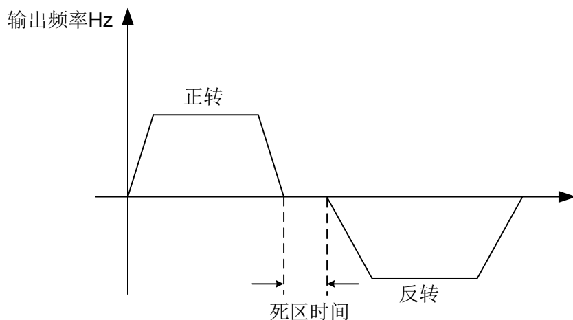
图 5-16 正反转死区时间示意图
