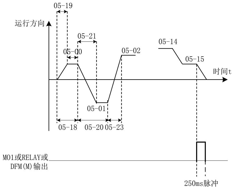
图 5-11 简易 PLC 示意图
