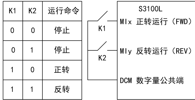
图 5-7 两线式模式 2
