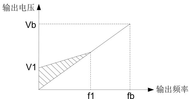
图 5-3 手动转矩提升示意图
