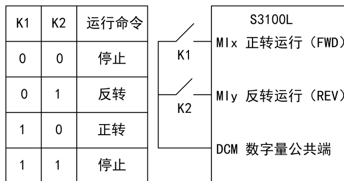
图 5-6 两线式模式 1
