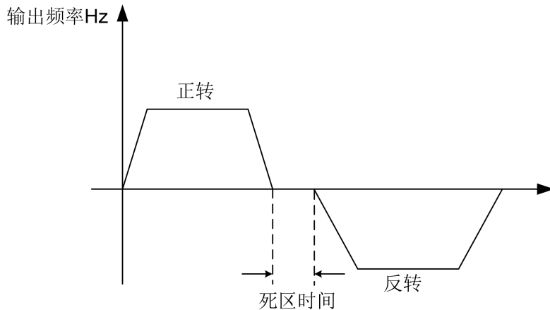
图 5-16 正反转死区时间示意图
