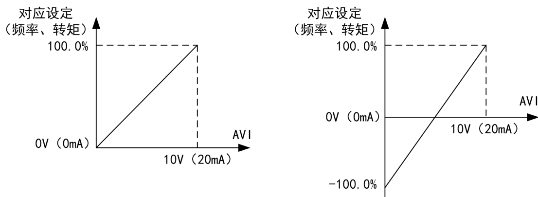
图 5-10 模拟给定与设定量的对应关系
