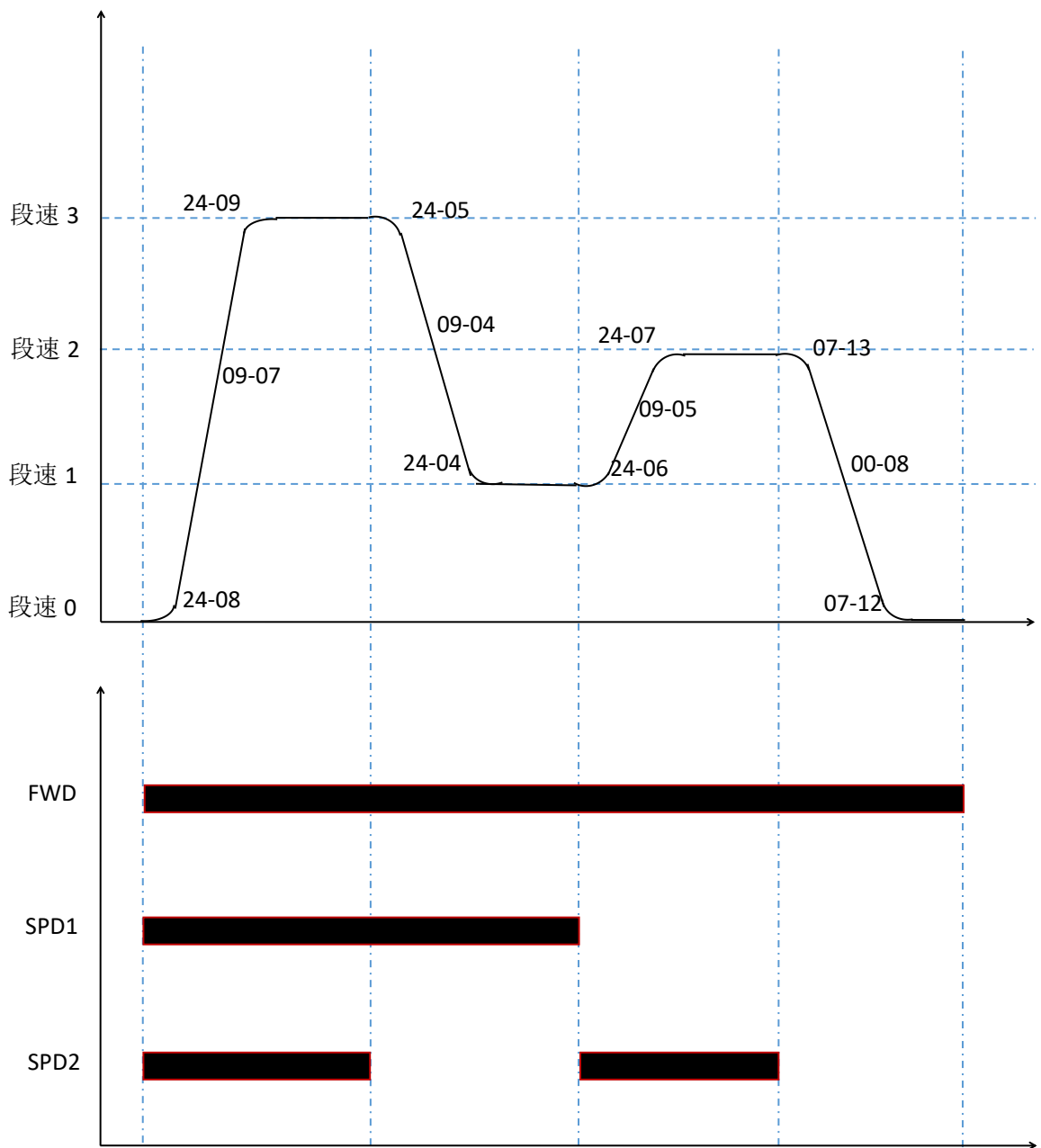
图 5-11 多段速相关参数示意图
