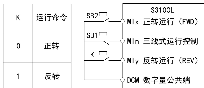
图 5-9 三线式控制模式 2
