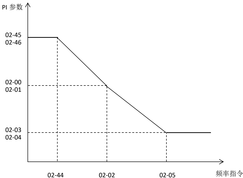
图 5-3 3 段式 PI 参数示意图
