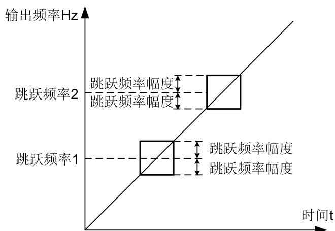
图 5-15 跳跃频率示意图
