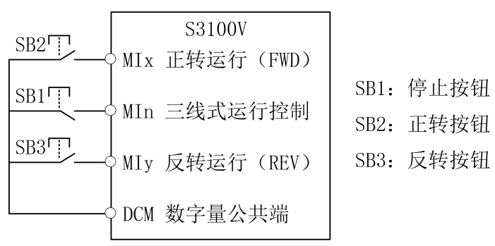
图 5-8 三线式控制模式 1
