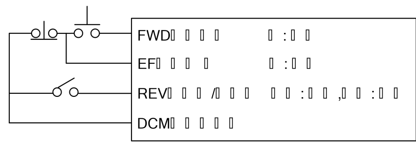
三线式控制（1）
