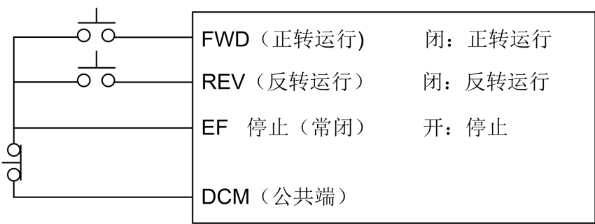
三线式控制（2）
