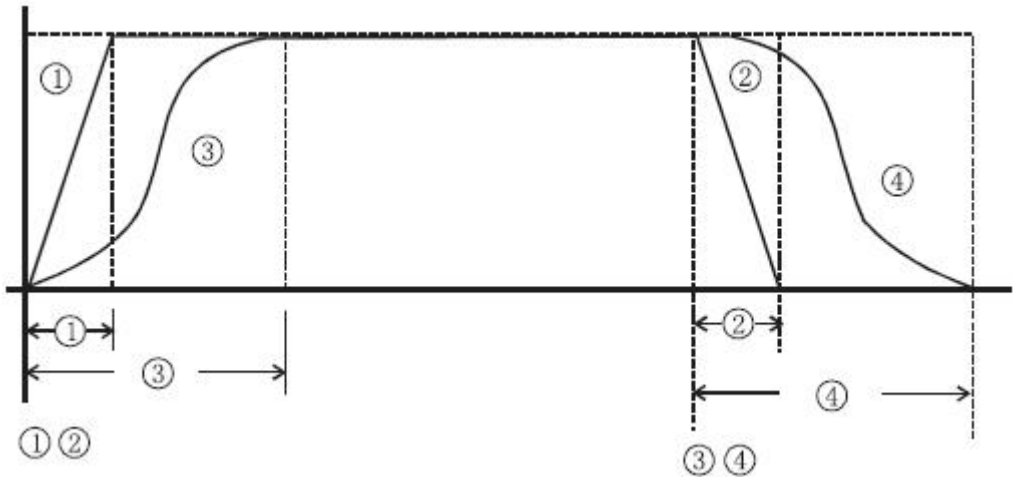
无 S 曲线时之加/减特性
