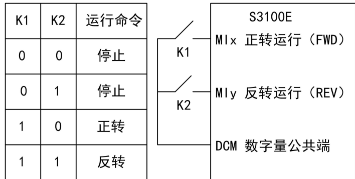
图 5-7 两线式模式 2
