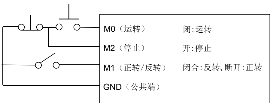
三线式控制（1）
