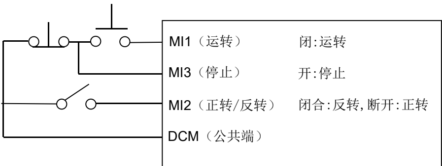
三线式控制（1）
