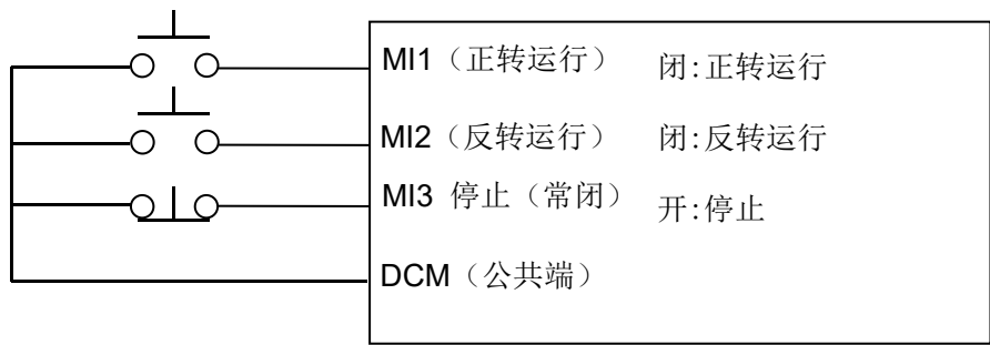
三线式控制（2）
