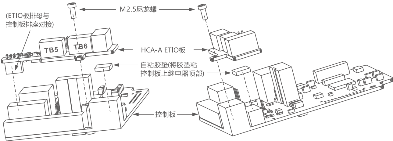
▪ 安装示意图
