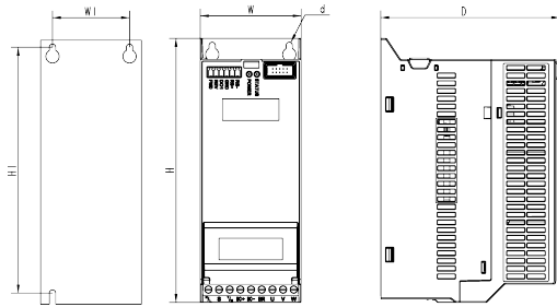
D1 Power unit size
