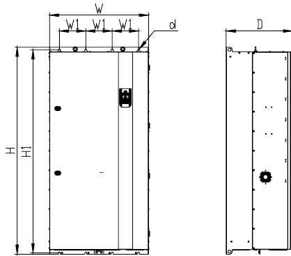
D10 Complete inverter size
